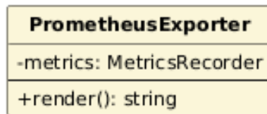
Figura 88: Classe — PrometheusExporter
