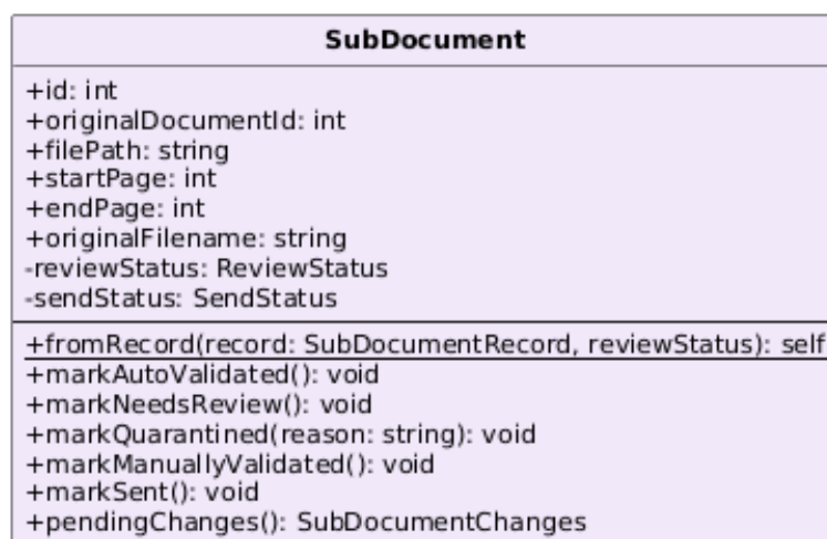
Figura 19: Classe — SubDocument
