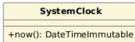
Figura 83: Classe — SystemClock
